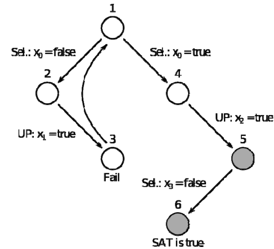
Рис. 3: Пример работы алгоритма DPLL. Метки Sel. и UP обозначены присваивания, происходящие на шагах выбора переменной и распространения «единичных» конъюнктов, соответственно.
