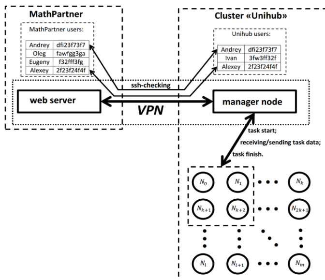
Рис. 1. Общая схема взаимодействия web-сервиса MathPartner и кластера Unihub.
