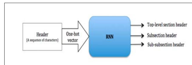
Рис. 1. Вход и выход классификатора заголовков Fig. 1. Input and output of the section classifier
