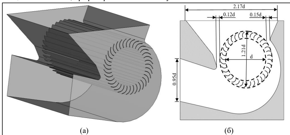
Рис. 1. Геометрия расчетной области: пространственная модель (а) и расчетная область (б)
