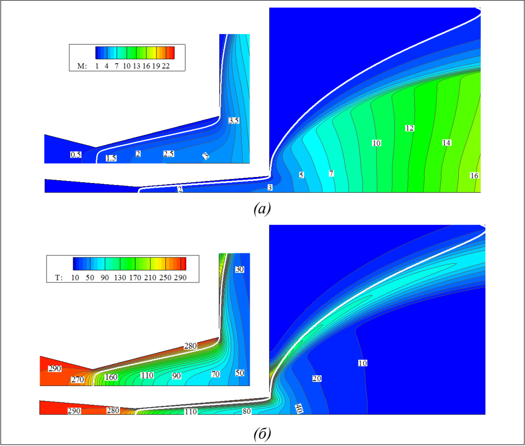
Рис. 3. Распределение числа Маха (а) и температуры (б) однофазного потока Fig. 3. Mach number distribution (a) and temperature field (b) for single phase flow
