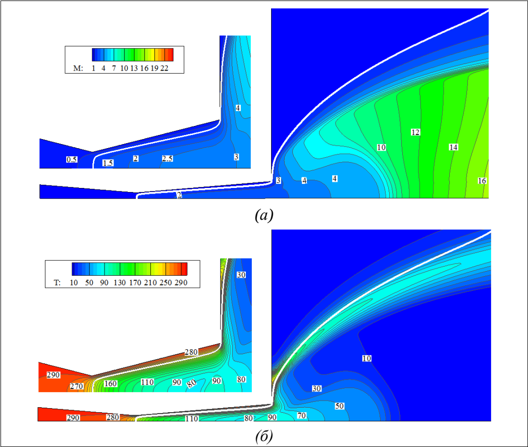
Рис. 5. Распределение числа Маха (а) и температуры (б) двухфазного потока Fig. 5. Mach number distribution (a) and temperature field (b) for two phase flow
