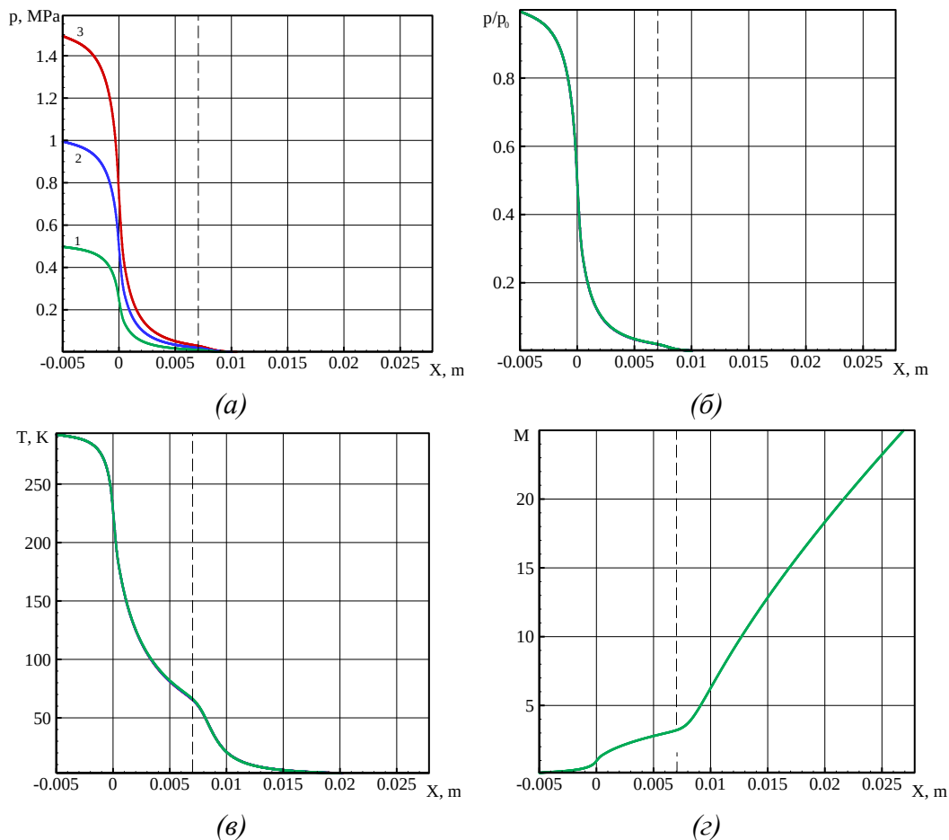
Рис. 4. Изменение статического (а) и относительного (б) давления, температуры (в) и числа Маха (г) вдоль оси Fig. 4. Variation of static (a) and dimensionless (b) pressure, temperature (c) and Mach number (d) along axis
