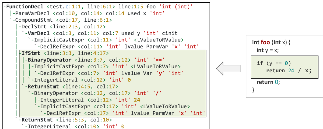
Листинг 2. Пример AST представления для кода на языке C. Listing 2. AST representation of function written in C language.
