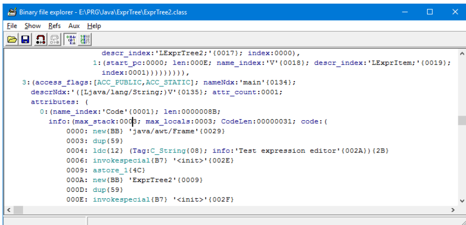
Рис. 3. Окно программы BinExpl при разборе файла класса Java
