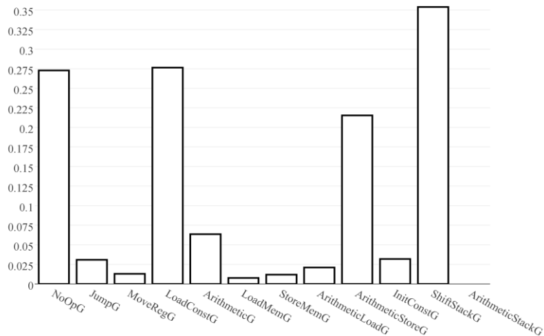
Рис. 3. Отношение числа классифицированных гаджетов данного типа к общему числу найденных гаджетов для архитектуры x86-64
