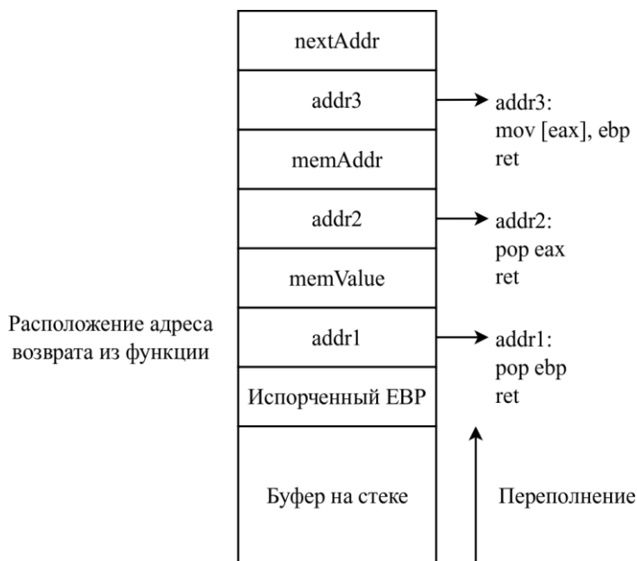
Рис. 1. Состояние стека после размещения ROP-цепочки, которая записывает значение memValue по адресу memAddr и передает управление на nextAddr
