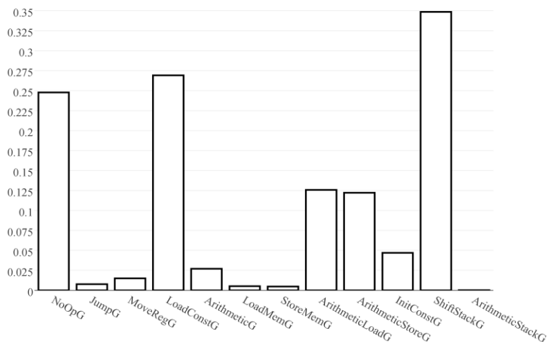
Рис. 2. Отношение числа классифицированных гаджетов данного типа к общему числу найденных гаджетов для архитектуры x86
