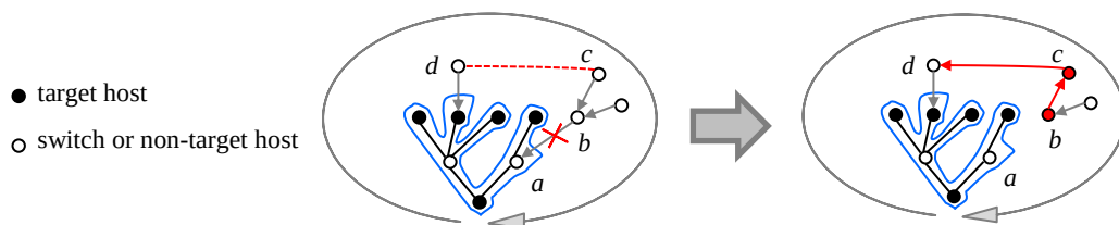
Рис. 9. Удаление ребра на дереве нецелевых хостов.
