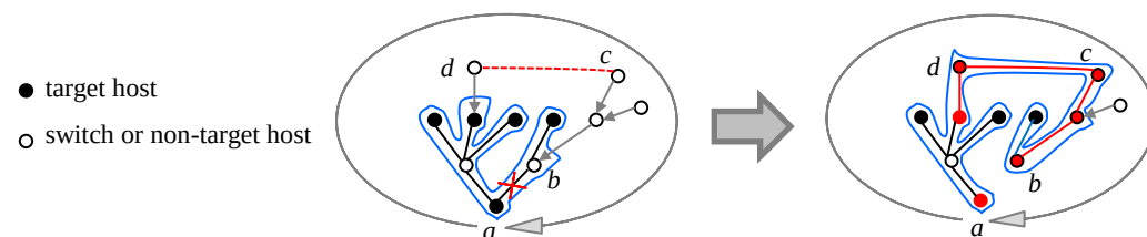
Рис. 10. Удаление ребра на дереве целевых хостов.
