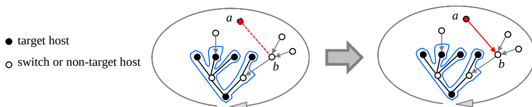
Рис. 11. Добавление одного коммутатора или нецелевого хоста и одного ребра, соединяющего его со «старой» вершиной графа.
