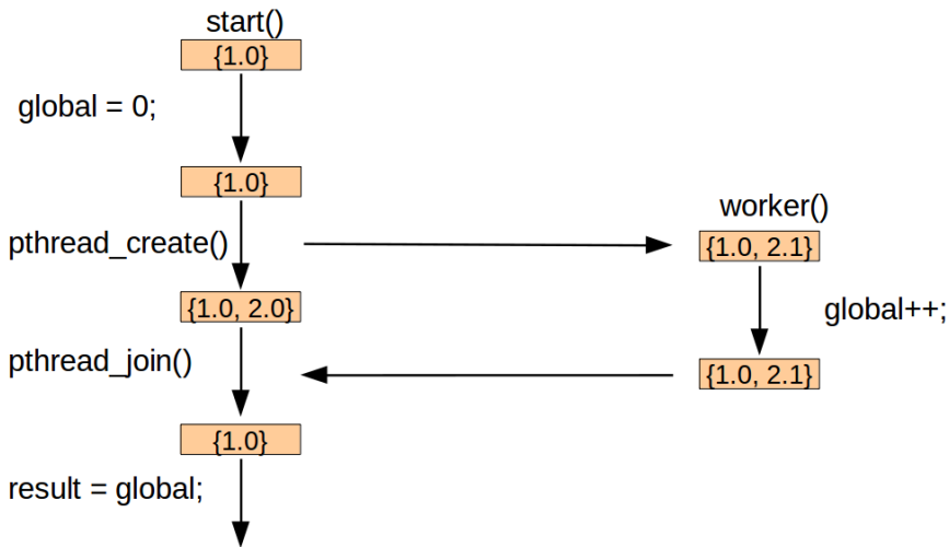
Рис. 6. Пример состояний анализа потоков
