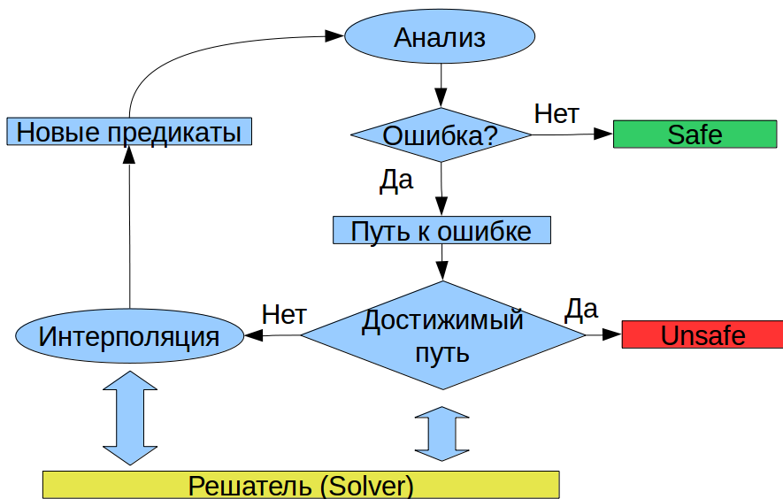
Рис. 3. Схема традиционного метода CEGAR
