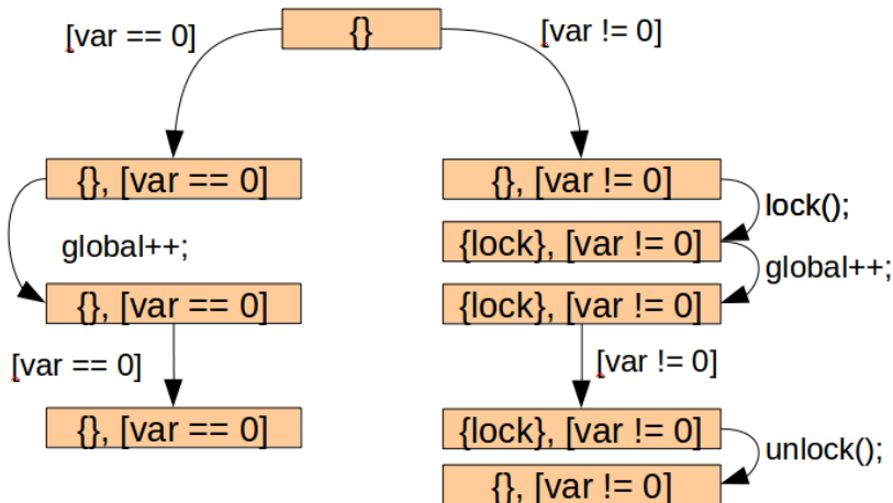
Рис 4. Пример анализа предикатов совместно с анализом примитивов синхронизации
