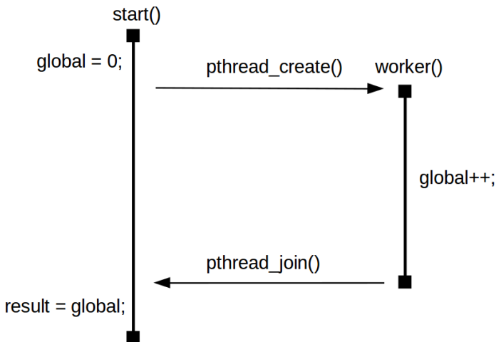
Рис. 5. Схема параллельной работы функций
