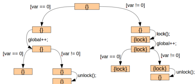
Рис. 1. Пример анализа примитивов синхронизации
