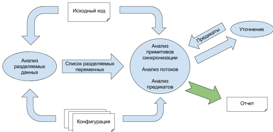
Рис. 2. Схема реализации метода
