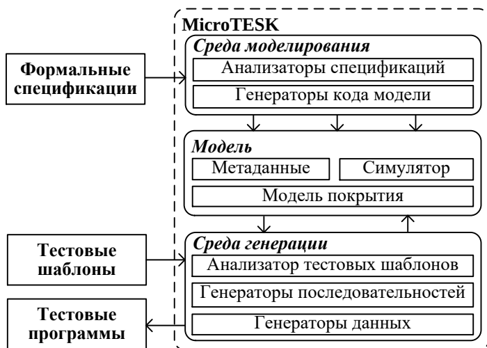
Рис. 1. Архитектура инструмента MicroTESK
