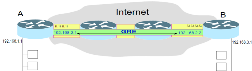
Рис. 1. Пример организации GRE-туннеля
