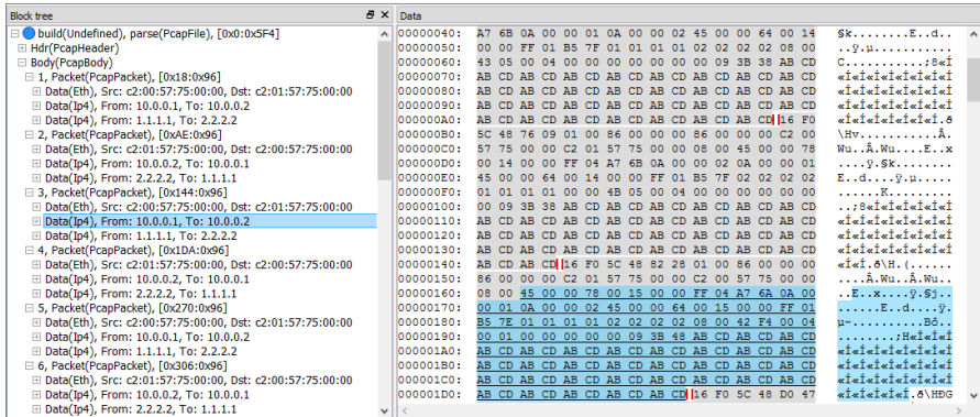
Рис. 3. Пример отображения стека протоколов для нескольких пакетов.
