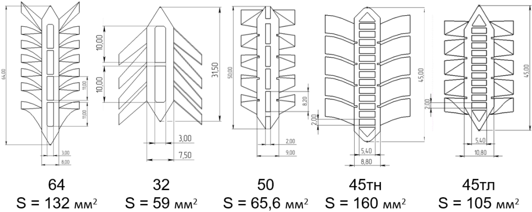
Рис. 1. Геометрия и размеры алюминиевых профилей, используемых в исследовании. Fig. 1. Geometry and dimensions of the aluminum profiles used in the study.
