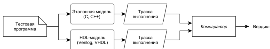
Рис. 1. Тестирование посредством сравнения трасс
