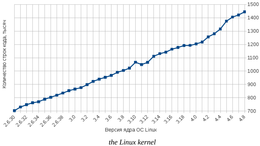
Рис. 4. Количество строк кода на языке программирования Си и языке ассемблера в ядре ОС Linux
