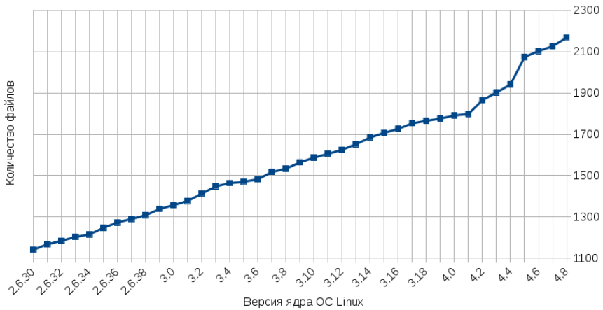
Рис. 3. Количество файлов на языке программирования Си и языке ассемблера в ядре ОС Linux
