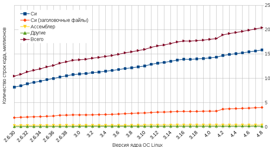
Рис. 2. Количество строк кода на различных языках программирования в ядре ОС Linux вместе с поставляемыми с ним загружаемыми модулями
