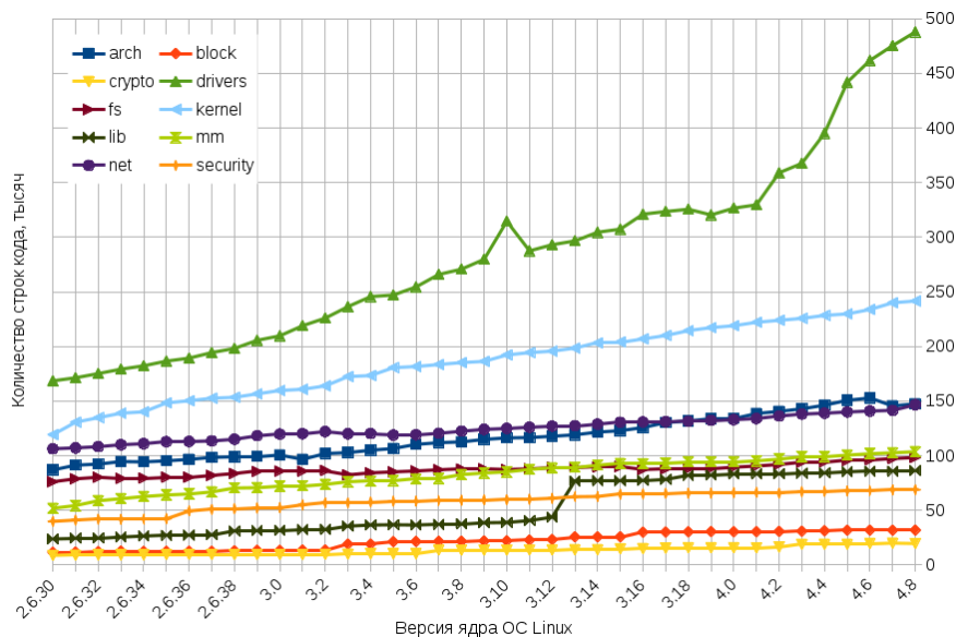
Рис. 6. Количество строк кода на языке программирования Си и языке ассемблера в основных подсистемах ядра ОС Linux
