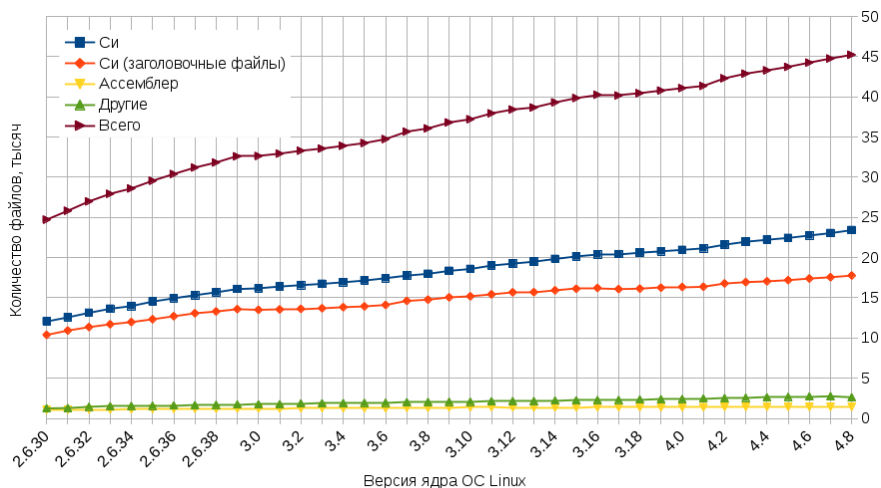
Рис. 1. Количество файлов на различных языках программирования в ядре ОС Linux вместе с поставляемыми с ним загружаемыми модулями
