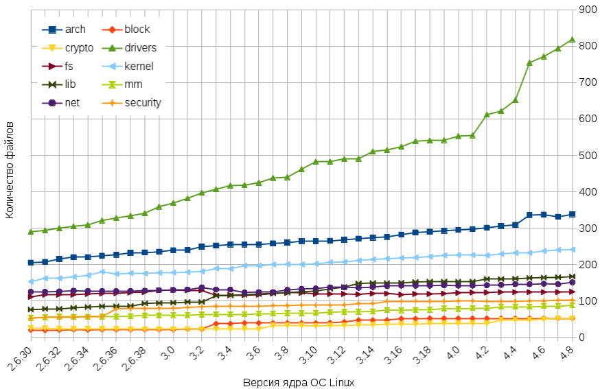
Рис. 5. Количество файлов на языке программирования Си и языке ассемблера в основных подсистемах ядра ОС Linux
