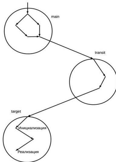
Рис. 3. Граф достижения точки инициализации дефекта Fig. 3. The graph of reaching a point of defect initialization
