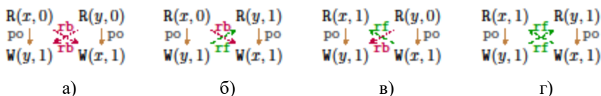
Рис. 1. Возможные исполнения программы LB в модели ARMv8.3 Fig. 1. Executions of program LB , which are allowed by model ARMv8.3
