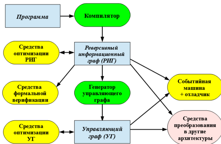
Рис. 4. Состав инструментальных средств, поддерживающих функционально-поточковое параллельное программирование
