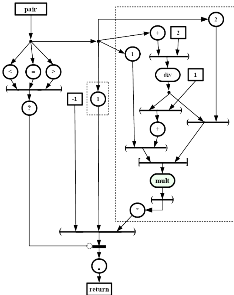
Рис. 3. Графическое представление функции перемножения в заданном диапазоне положительных чисел
