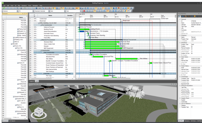
Рис. 2. Главное окно графического интерфейса пользователя системы Synchro.
