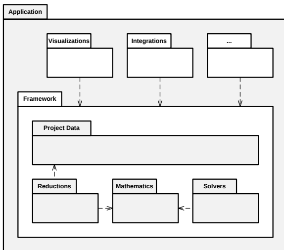
Рис. 1. Организация объектно-ориентированного каркаса для разработки приложений теории расписаний.
