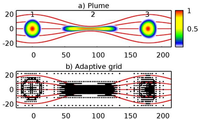
Рис. 6 Движение облака примесей (а) и эволюция соответствующей адаптивной сетки (б) в сужающемся-расширяющемся потоке для различных моментов времени (1), (2), (3).
