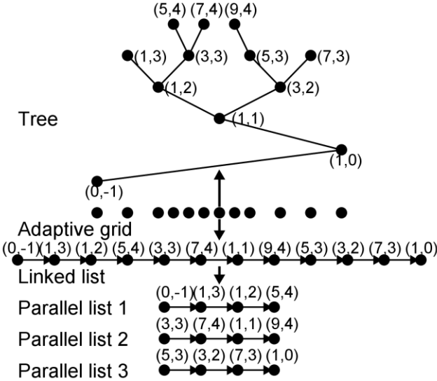
Рис. 3 Представление адаптивной сетки в виде дерева и связного списка.
