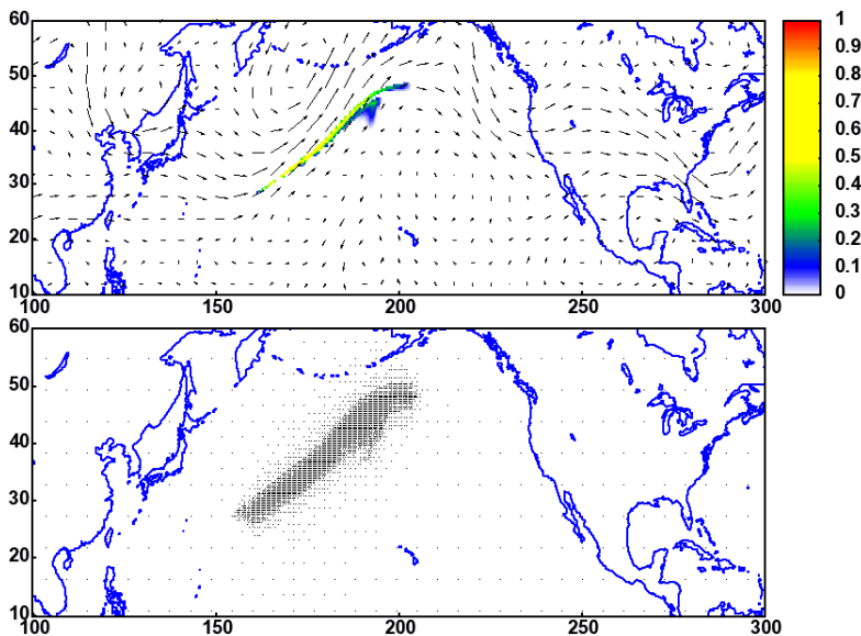
Рис. 7 Перенос облака примесей над Тихим океаном 1-ого мая 2001 года (верхняя панель) и соответствующая адаптивная сетка (нижняя панель).
