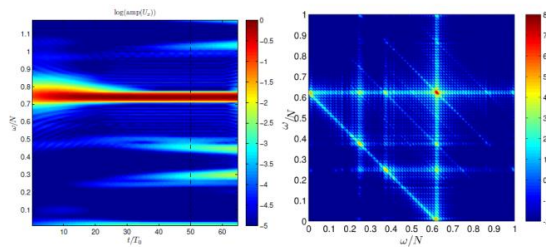
Рис. 5: Частотно-временная диаграмма и биспектр для слабонеустойчивого аттрактора
