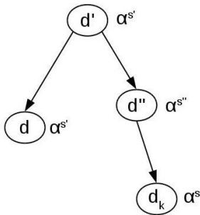
Рис. 5. Иллюстрация распределения степеней \alpha в разных случаях Fig. 5 Distribution of degrees of \alpha in different cases.
