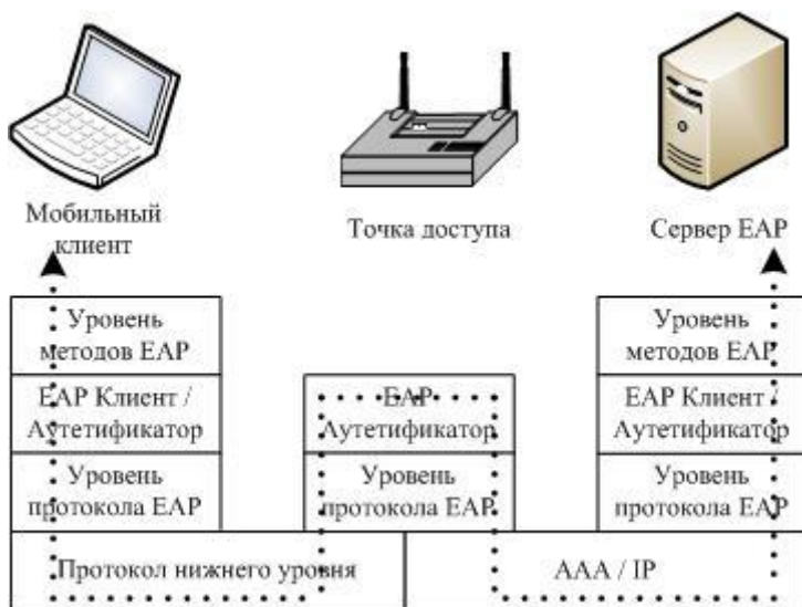
Рис. 2. Стеки протоколов EAP
