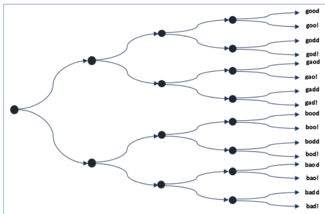
Рис. 2. Входные данные после каждой итерации алгоритма
