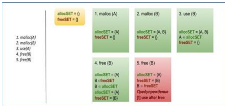
Рис. 6. Пример работы алгоритма
