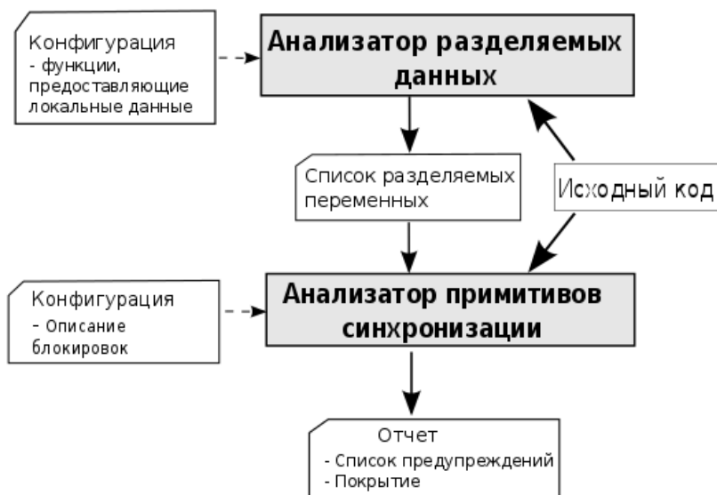
Рисунок 4 — Этапы CPA Lockator
