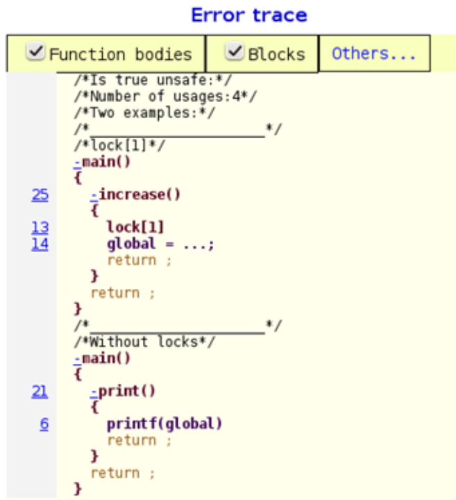
Рисунок 9 — Пример сообщения об ошибке. Трасса ошибки с точками захвата блокировок и точками вызова функций, каждая из которых ссылается на соответствующую строку исходного кода (см. рис. 8)
