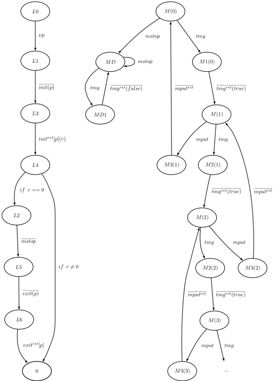
Рис. 4. Пример процесса P_{\text{module}} (слева) и процесса P_{\text{trymoduleget}} (справа)
