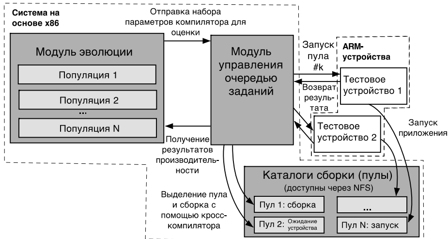
Рис 1. Компоненты ТАСТ и общая схема работы
