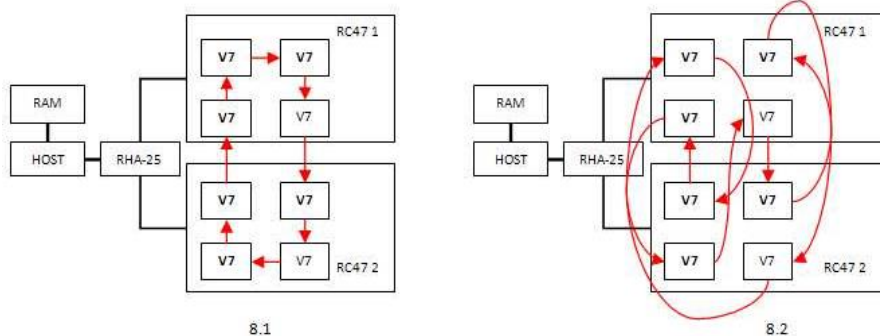
Рис. 7 Взаимодействие ПЛИС в случае 8ми одновременных передач
