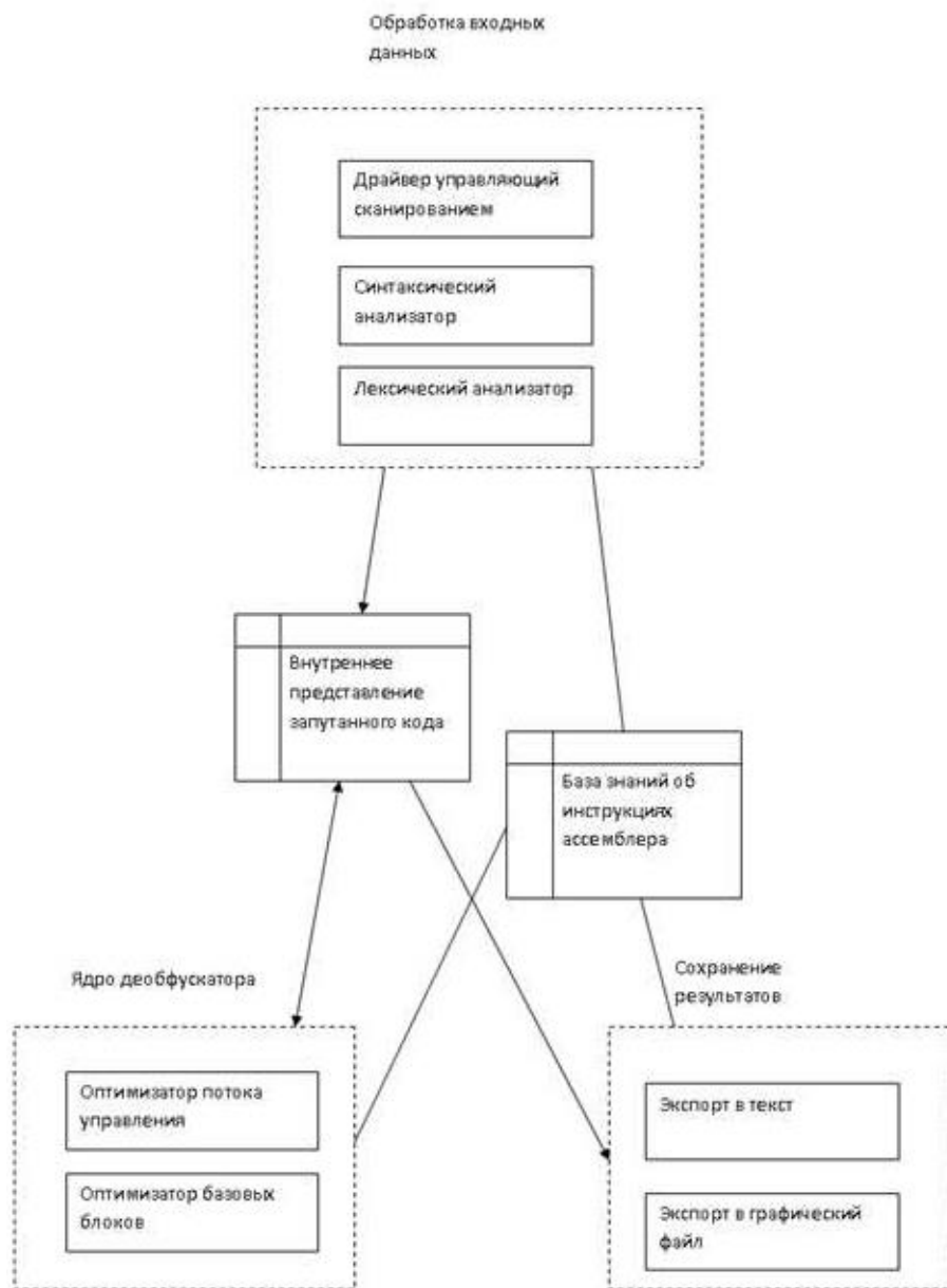
Рис.1. Архитектура системы
