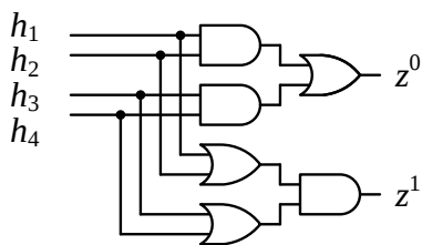
Рис. 8. Структурная схема 2/4-TSC Fig. 8. 2/4-TSC structural circuit
