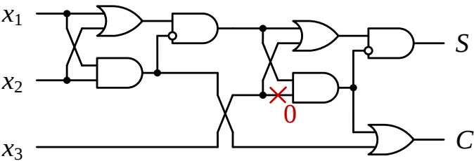
Рис. 1. Схема полного сумматора Fig. 1. Full-adder circuit
