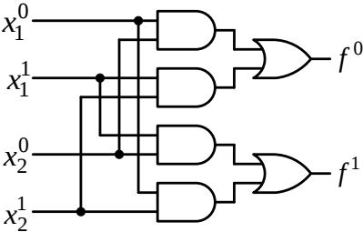
Рис. 5. Структурная схема TRC Fig. 5. TRC structural circuit
