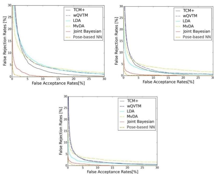
Рис. 3. Сравнение ROC-кривых различных методов для многокамерной задачи верификации на базе OULP для тестового угла 85^\circ и обучающих углов, равных 55^\circ , 65^\circ , and 75^\circ , соответственно
